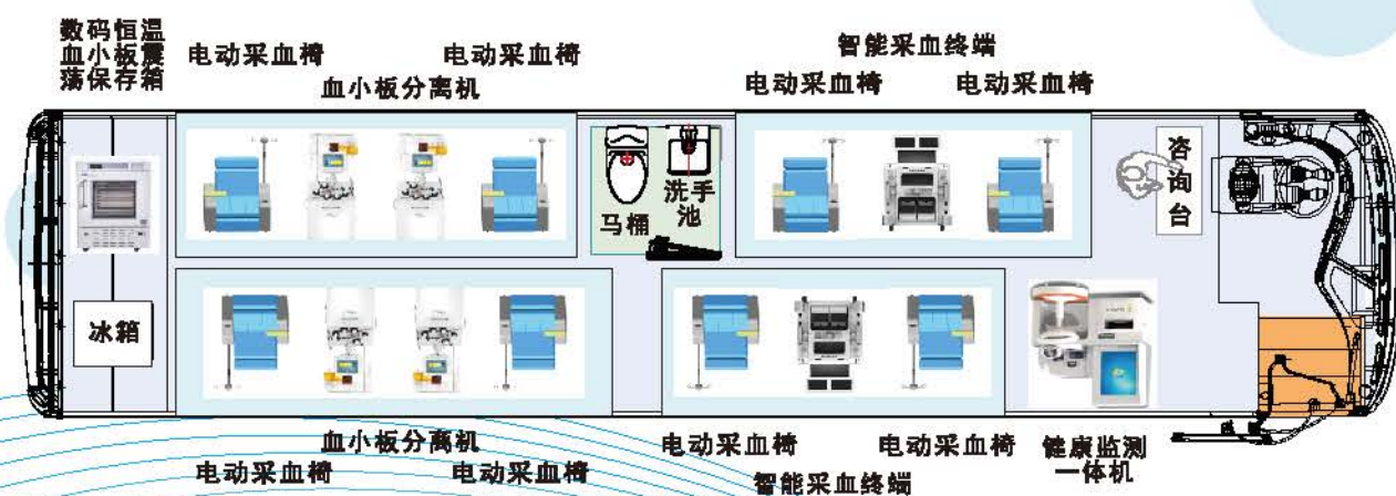
智能献血车平面布置图
