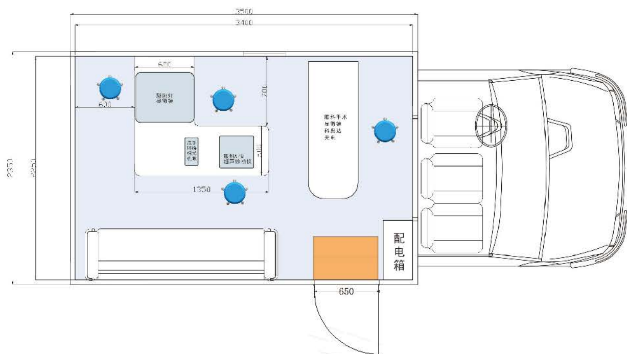
5995mm眼科体检车平面布置图
