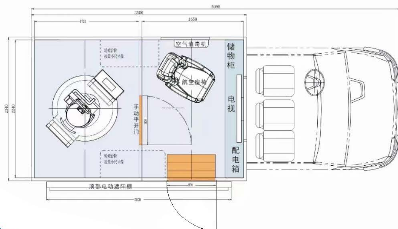
5995mm口腔宣教车平面布置图
