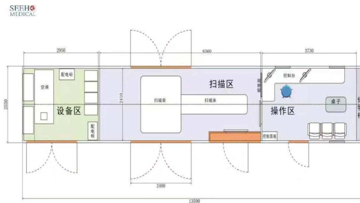
显浩磁共振车平面布局图
