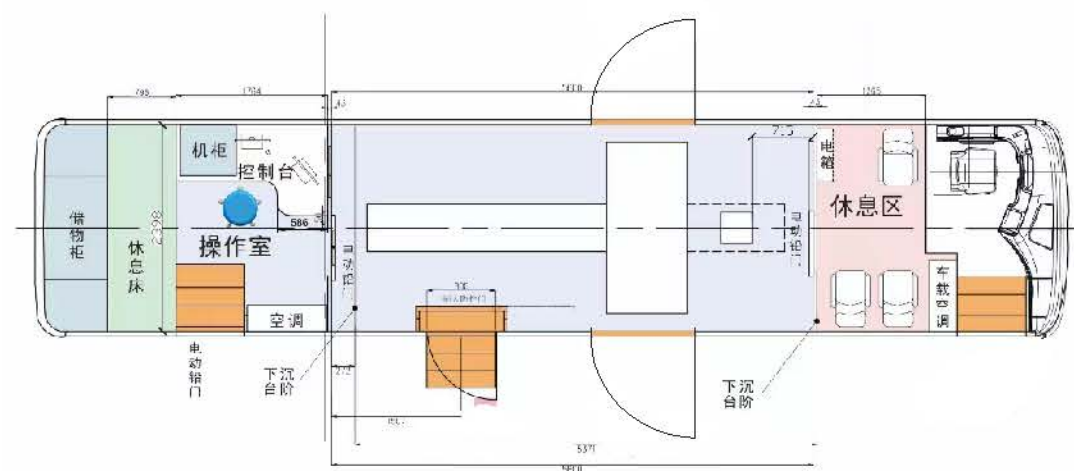
1200mmCT客车平面布置图
