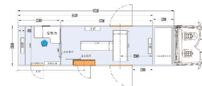
12000mm单轴CT带发电机组平面布置图
