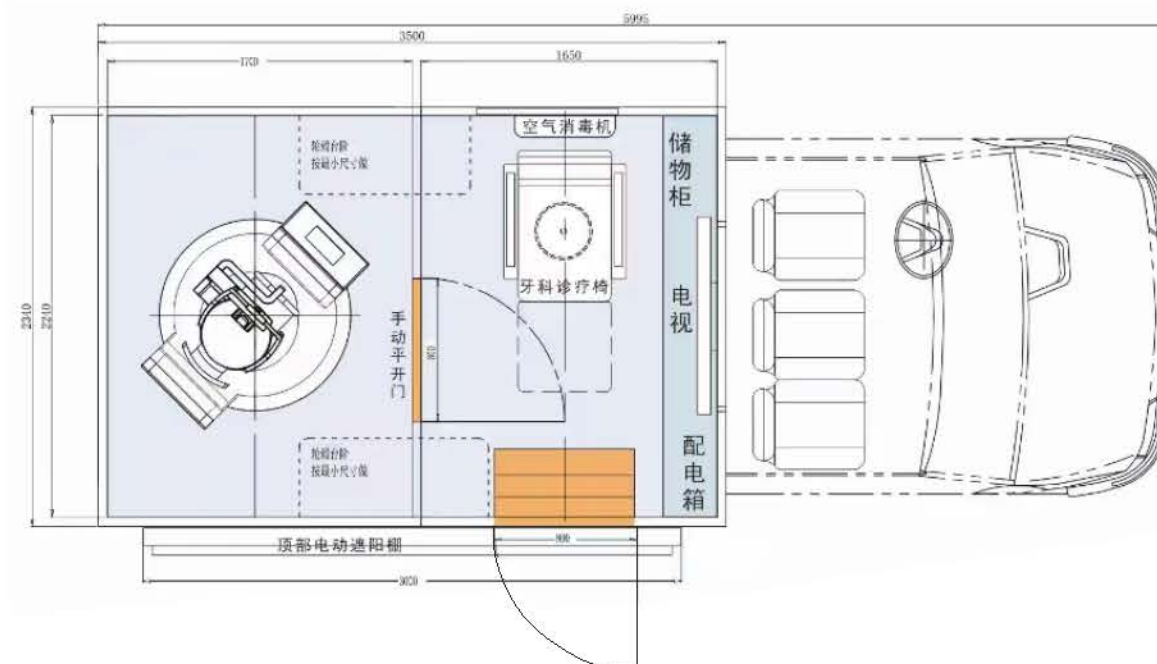
5995mm牙科诊疗车平面布置图
